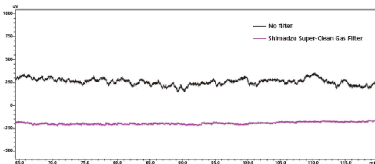
Рис.1 Эффект снижения шума базовой линии после установки газового фильтра.
